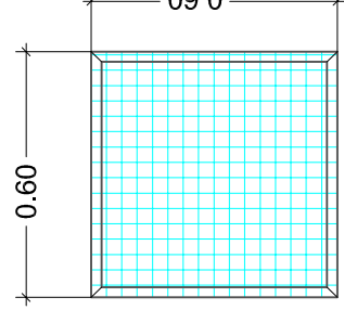
Gitterrost Winkelisen 25x25x5
