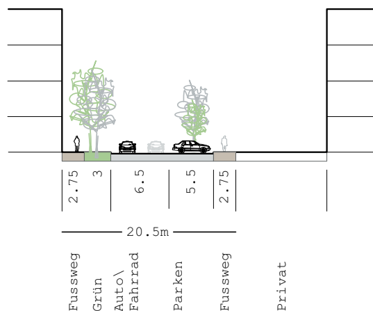
Straßenprofil
