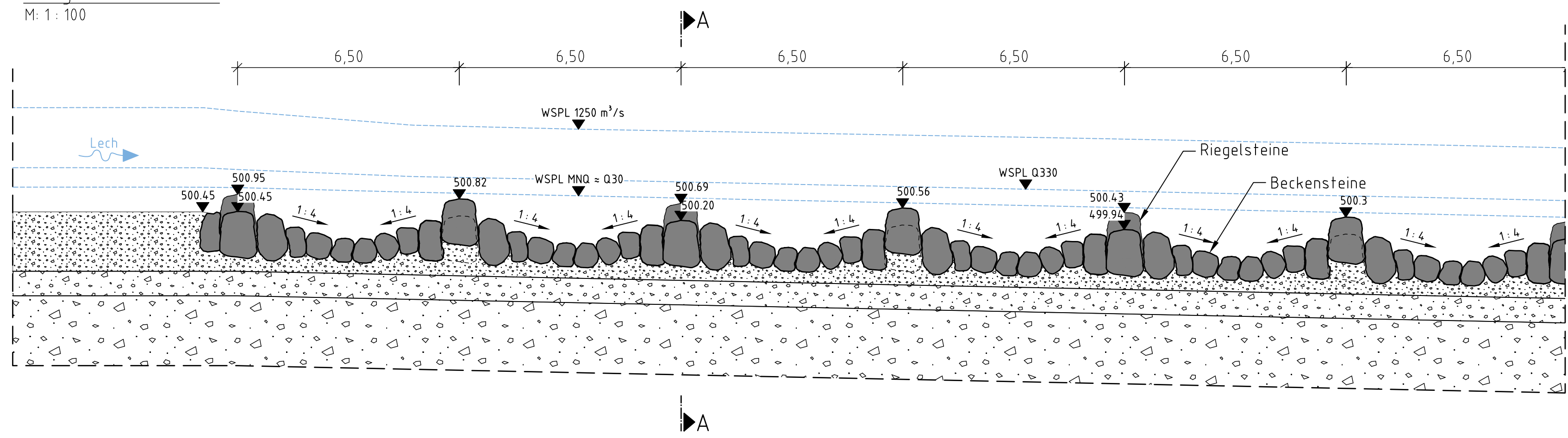
Längsschnitt B - B M: 1: 100
