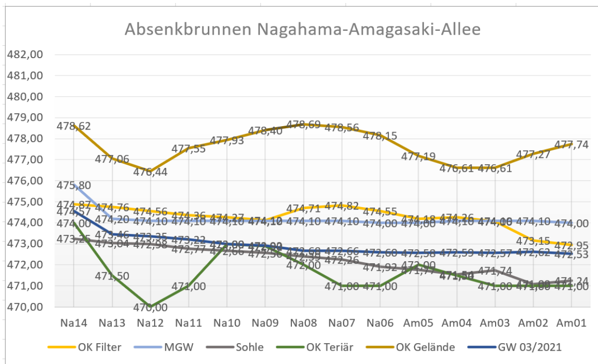
Abb. 2: Höhenlage der Brunnen in Nagahama- und Amagasaki-Allee
