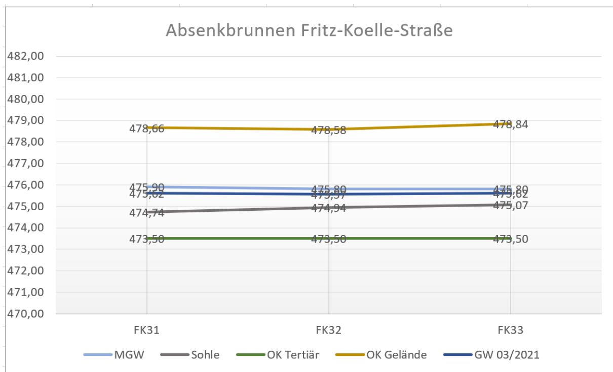
Abb. 4: Höhenlage der Brunnen in der Fritz-Koelle-Straße
