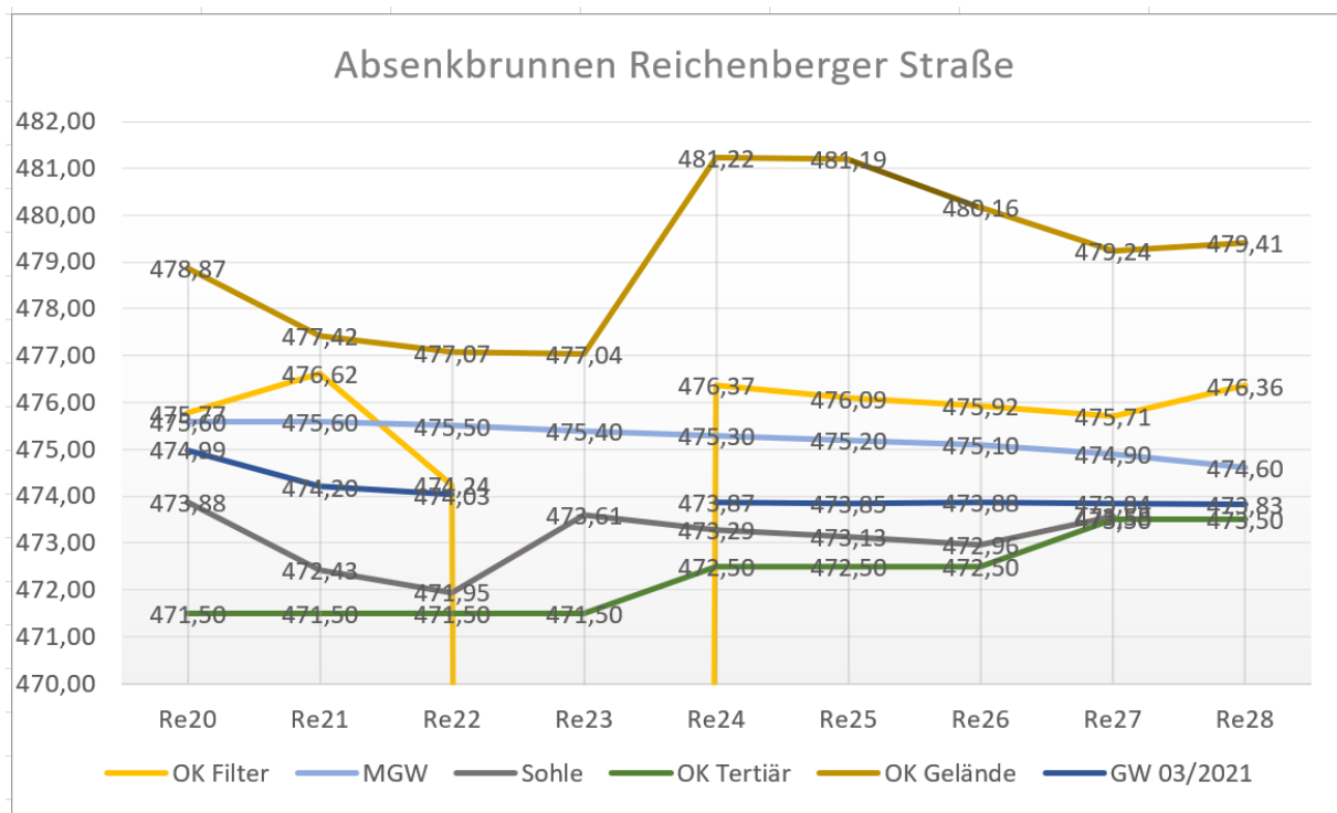
Abb. 3: Höhenlage der Brunnen in der Reichenberger Straße (Re23 wurde überbaut, daher konnten die Oberkante der Filterstrecke und der Gw-Spiegel nicht ermittelt werden)
