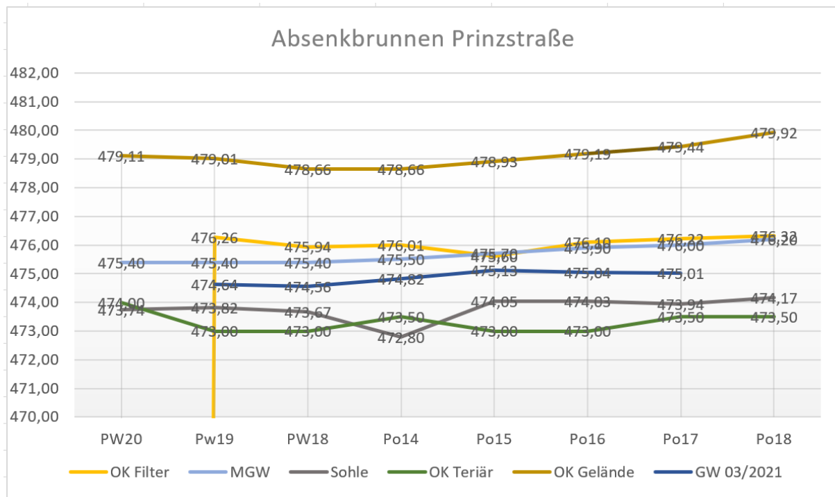
Abb. 1: Höhenlage der Brunnen in der Prinzstraße (Auf Grund seiner baulichen Ausführung konnten die Oberkante der Filterstrecke und der GW-Spiegel in Pw20 nicht ermittelt werden)
