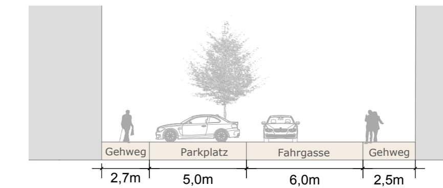
Schnitt B-B M 1:200
