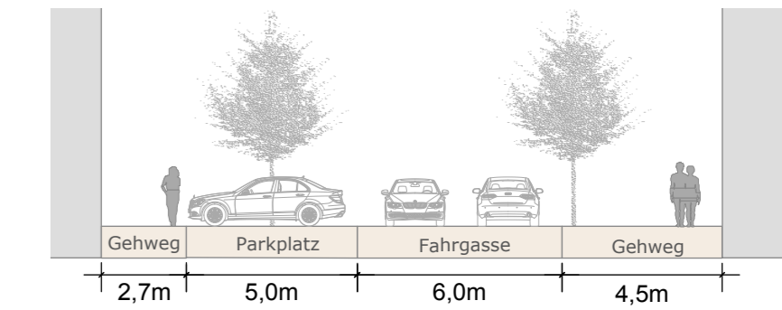
Schnitt A-A M 1:200
