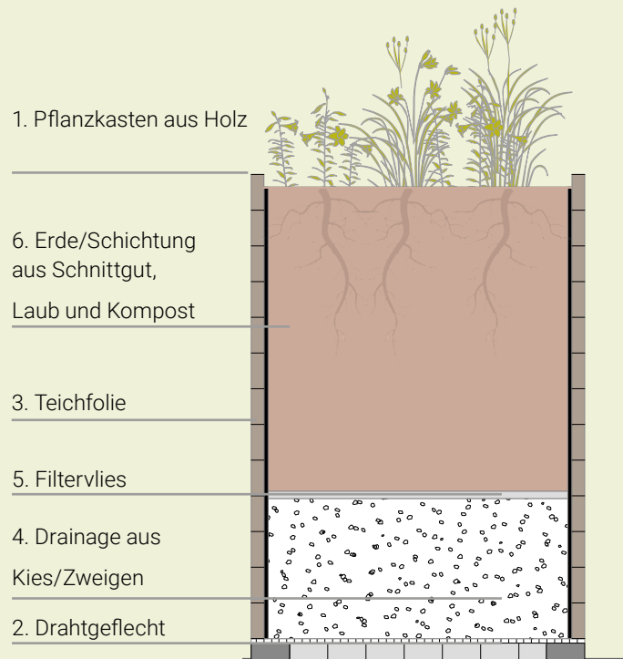
Schematische Darstellung Aufbau Hochbeet
