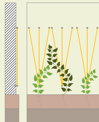
Berankung mit Seilen z. B. aus Polypropylen
